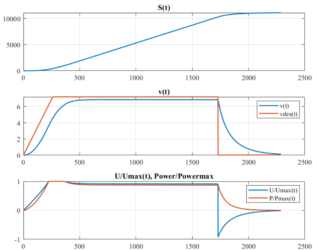
Рисунок 16 – Воздействие в виде течения во встречном направлении
