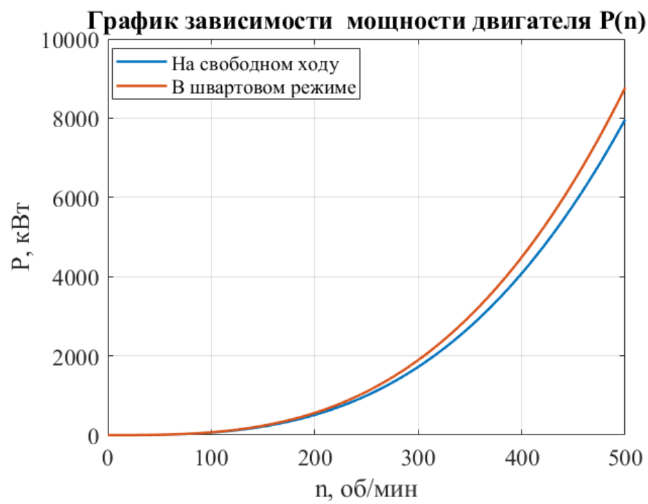
Рисунок 3 – График зависимости мощности двигателя от оборотов в разных режимах
