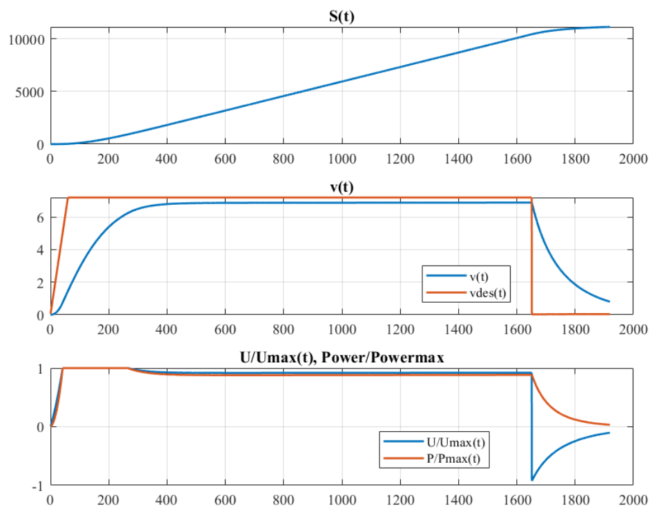
Рисунок 7 – Результат моделирования t_l = 60 ; S_2 = 700
