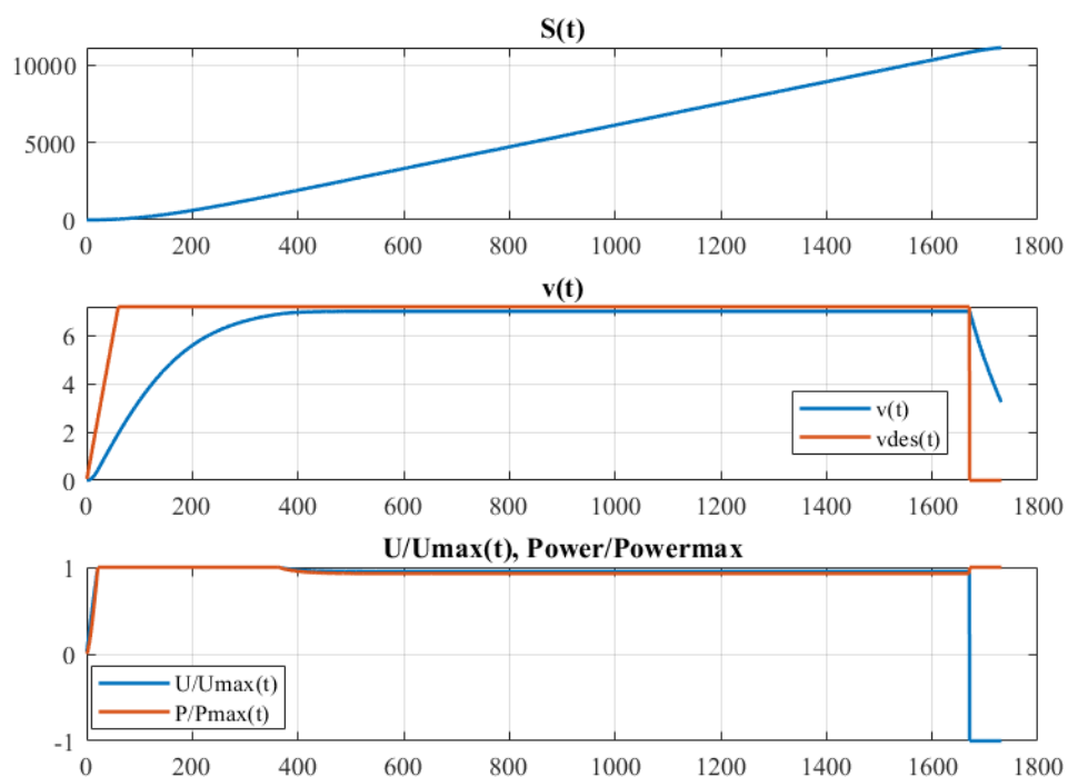
Рисунок 5 – Результат моделирования при a_V = 25
