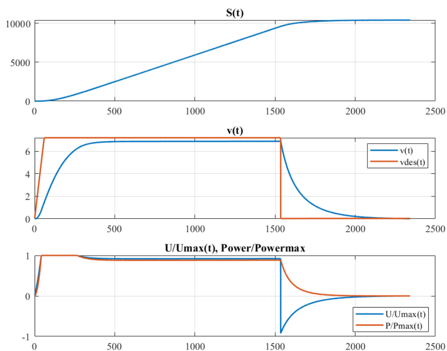
Рисунок 8 – Результат моделирования t_l = 60 ; S_2 = 1500
