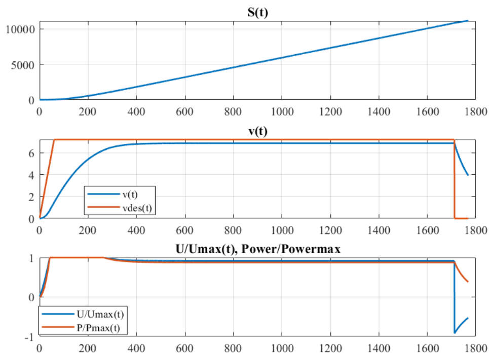
Рисунок 4 – Результат моделирования при a_V = 8
