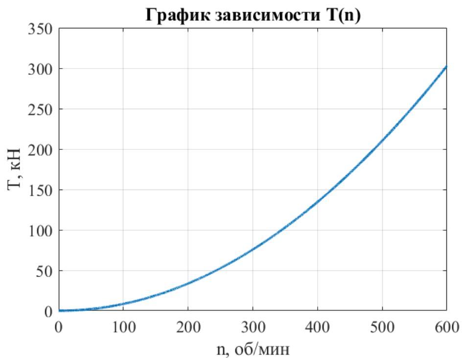
Рисунок 2 – График зависимости тяги от оборотов на свободном ходу.
