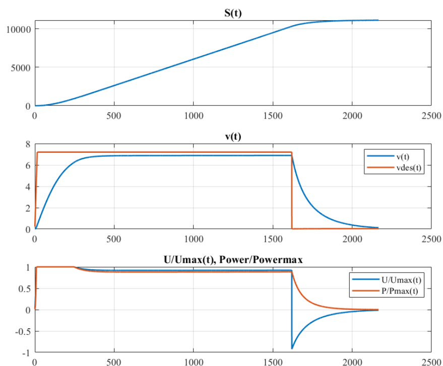
Рисунок 10 – Результат моделирования t_l = 15 ; S_2 = 800
