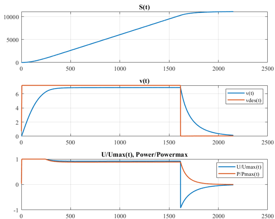
Рисунок 11 – Результат моделирования t_l = 5 ; S_2 = 800
