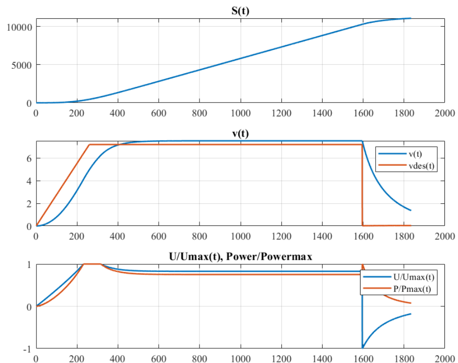
Рисунок 17 – Результат работы П-регулятора с попутным течением
