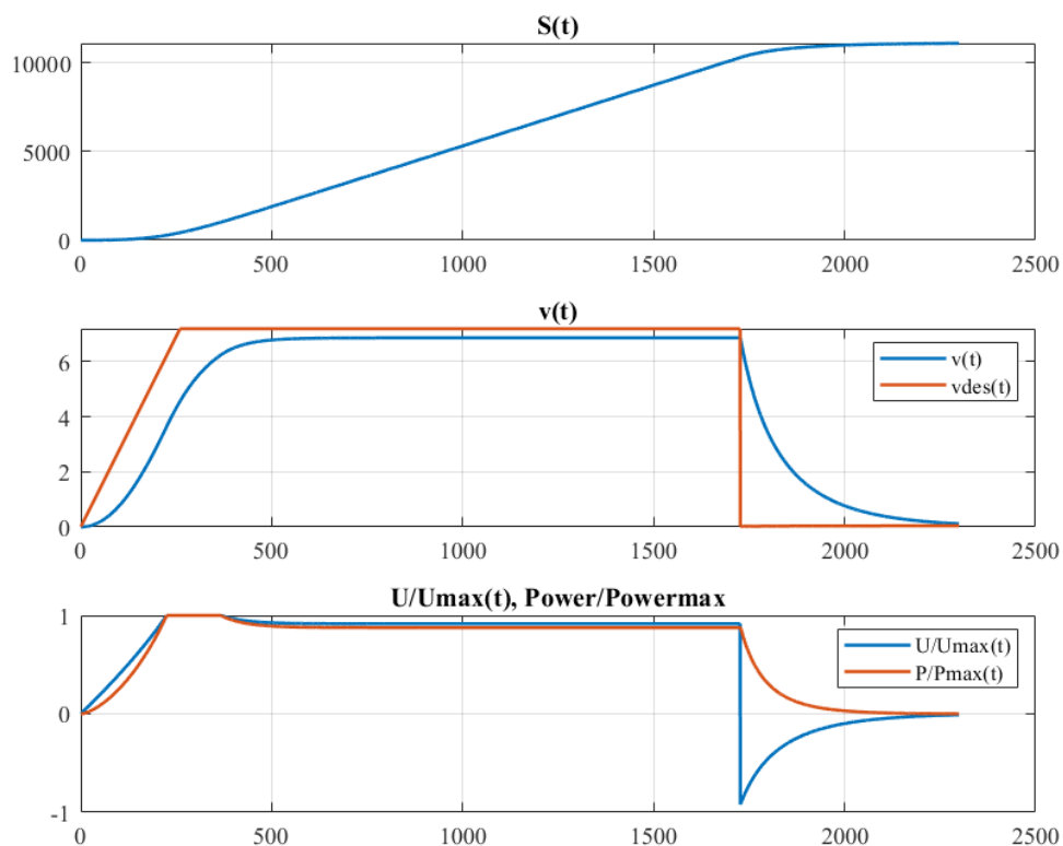
Рисунок 18 – Результат работы П-регулятора с встречным течением
