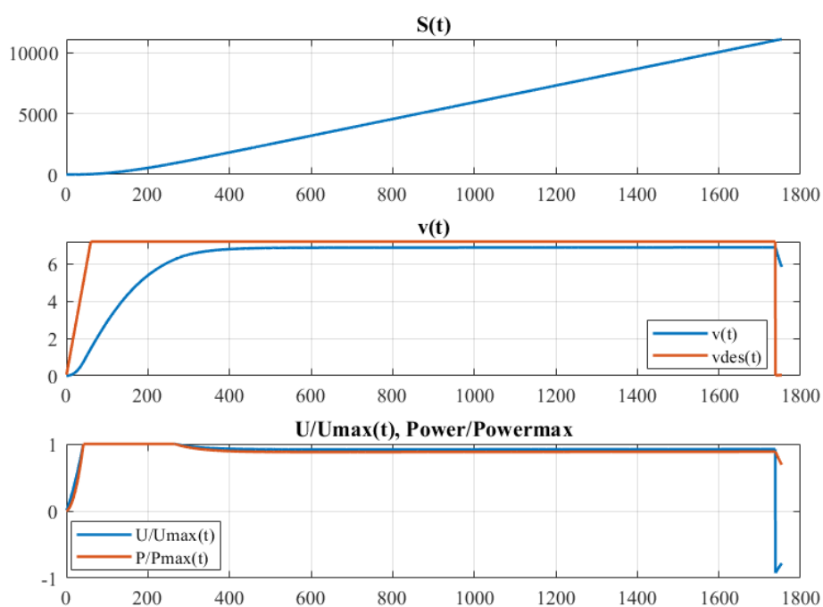
Рисунок 6 – Результат моделирования t_l = 60 ; S_2 = 100
