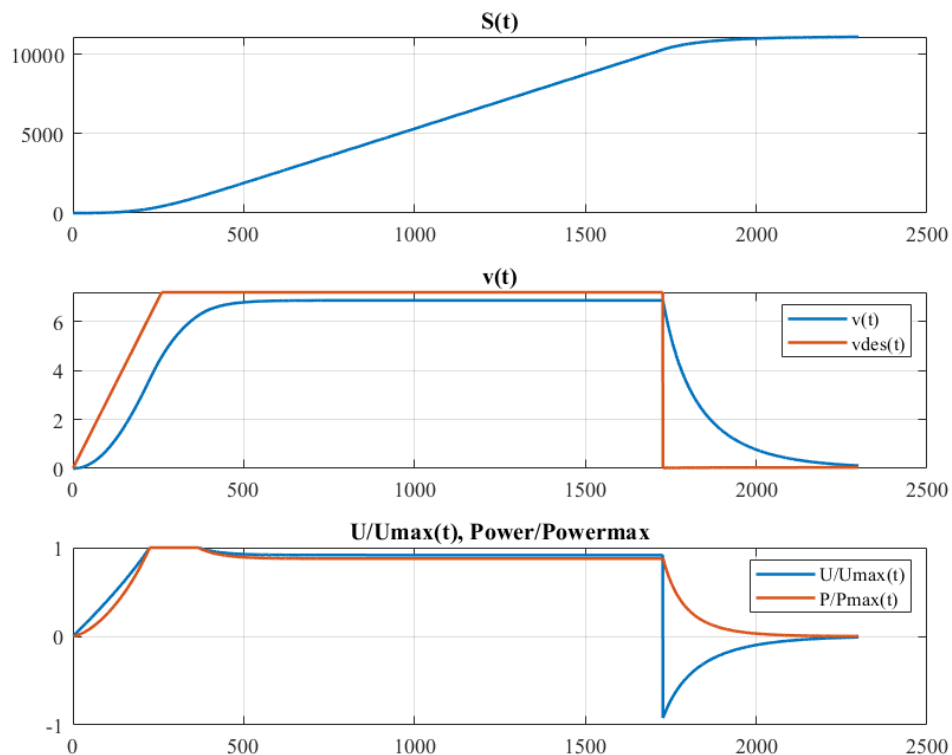
Рисунок 14 – Моделирование разгона и торможения судна при оптимальных параметрах
