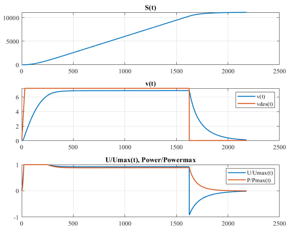
Рисунок 9 – Результат моделирования t_l = 30 ; S_2 = 800
