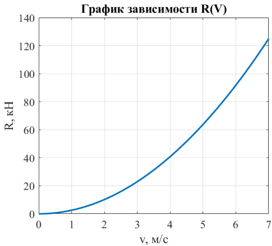
Рисунок 1 – График зависимости сопротивления движения от скорости.
